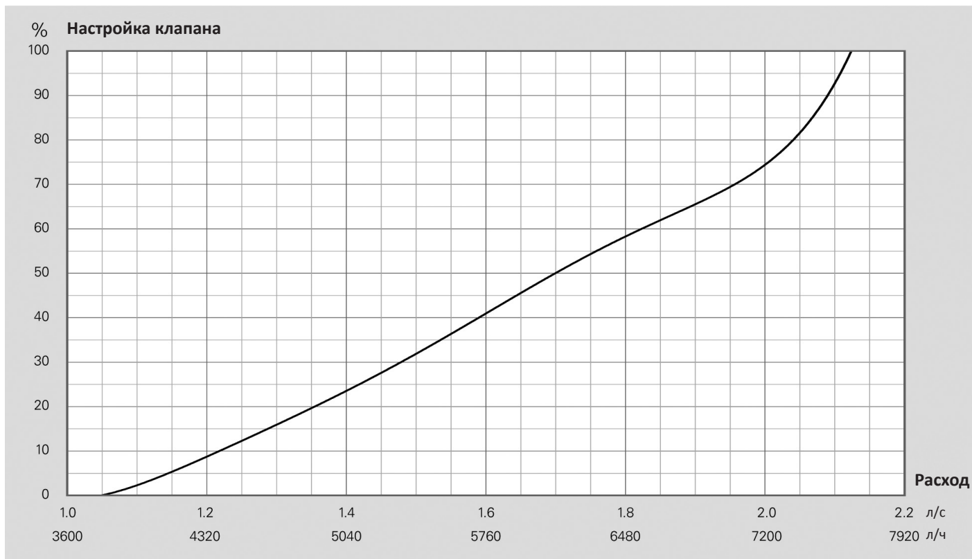
Номограмма расхода БРОЕН DYNAMIC DN 040S:
