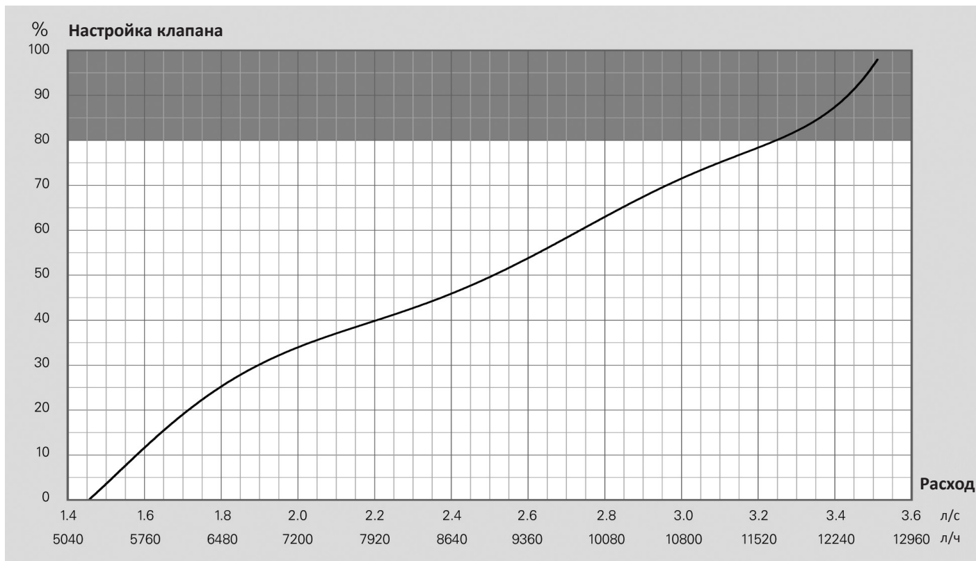
Номограмма расхода БРОЕН DYNAMIC DN 050H:
